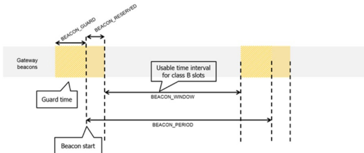
图 12：信标时序
